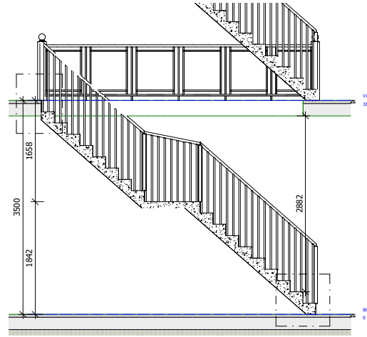
1 | Doorsnede met beuging en trapleuning 1 : 10
