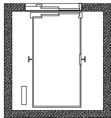
2 | Bovenaanzicht 1 : 10
