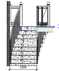
6 | Doorsnede detail 1 : 10
