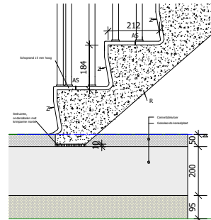
3 | Onder detail 1 : 5
