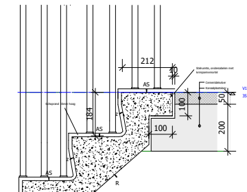
4 | Boven detail 1 : 5
