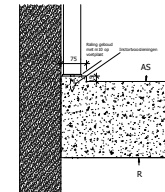
7 | Doorsnede detail 1 : 10
